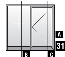
One sash door with fixed panel outwards opening with threshold Μονόφυλλη ανοιγόμενη πόρτα με ένα σταθερό- ανοιγόμενη έξω με κατωκάσι
