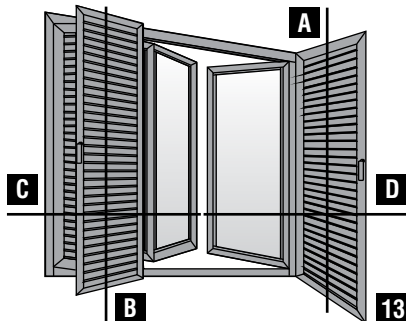
Τρίφυλλο ανοιγόμενο - ανακλινόμενο παράθυρο με παντζούρι Three sash tilt & turn window with shutter
