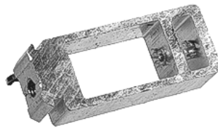
160 11 213 91 / inox βίδα Σύνδεσμος ταφ εσωτερικός | T-Connector Αλουμίνιο | Aluminum
