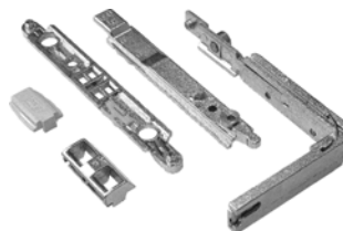
415 15 801 00 Βασικό σετ μηχανισμού - πλευρα χειρουλιου | Jet Ak8 locking parts for geared Ζάμακ | Zamak
