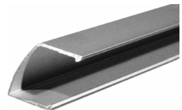
425 30 401 00 Καπακι ντιζας φεγγιτη | Cover for transom rod Αλουμινιο | Aluminium
