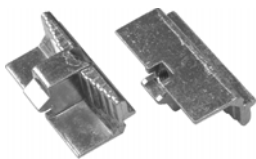
415 45 939 00 Πλακακι κλειδωματος συρτη ρυθμιζομενο(σετ) ; Shoot bolt locking plate adjustable (set) Ζάμακ ;Zamak
