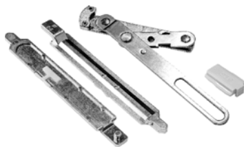
415 15 803 00 Συρτης εξωτερικος μονοκομματος ; Rebate shoot bolt Ζάμακ ;Zamak
