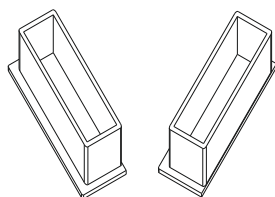
Τάπα στενού φύλλου S366 End cover for S366 narrow sash
