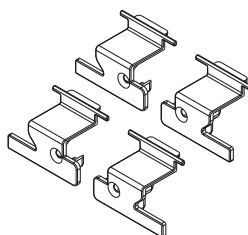
Τάπα μπινιού S358 End cover for S358 adjoining profile
