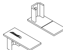
Ζεύγος ταπών για προφίλ ενίσχυσης M12412 Pair of end caps for stiffener profile M12412
