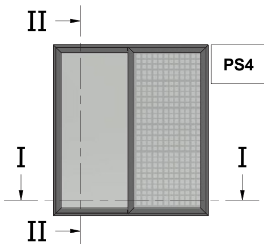
Two Sash Parallel Sliding Window 45 Degrees Cut with Flyscreen Δίφυλλο Επάλληλο Συρόμενο με κοπή 45 μοιρών με Σήτα
