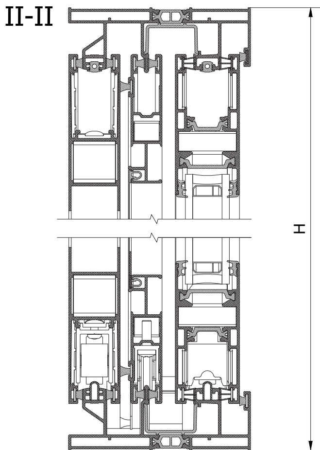
Μονόφυλλο Χωνευτό Συρόμενο με 45° κοπή με Σήτα και Παντζούρι Pocket Sliding 45° Cut with Flyscreen and Shutter
