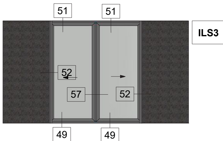
Pocket Sliding Window Meeting Stile 45 Degrees Cut with Shutter Χωνευτό Συρόμενο Φιλητό με κοπή 45 μοιρών και Παντζούρι
