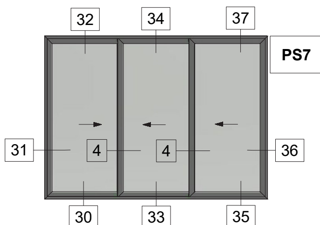
Three Sash Parallel Sliding Window 45 Degrees Cut Τρίφυλλο Επάλληλο Συρόμενο με κοπή 45 μοιρών
