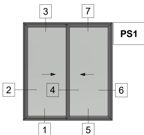
Two Sash Parallel Sliding Window 45 Degrees Cut Δίφυλλο Επάλληλο Συρόμενο με κοπή 45 μοιρών
