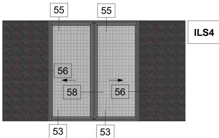
Pocket Sliding Window Meeting Stile 45 Degrees Cut with Flyscreen and Shutter Χωνευτό Συρόμενο Φιλητό με κοπή 45 μοιρών Σήτα και Παντζούρι
