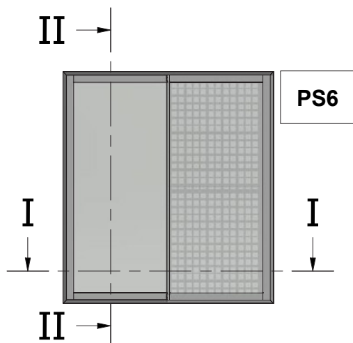
Two Sash Parallel Sliding Window 90 Degrees Cut with Narrow Interlock and Flyscreen Δίφυλλο Επάλληλο Συρόμενο με κοπή 90 μοιρών, Στενό Γάντζο και Σήτα
