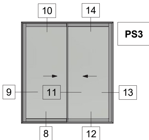
Two Sash Parallel Sliding Window 90 Degrees Cut with Narrow Interlock Δίφυλλο Επάλληλο Συρόμενο με Κοπή 90 Μοιρών και Στενό Γάντζο
