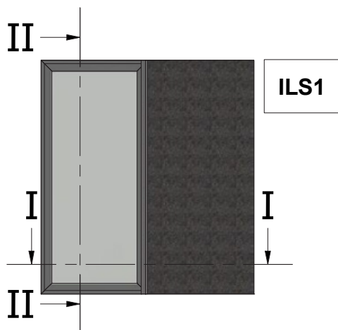
Μονόφυλλο Χωνευτό Συρόμενο με 45° κοπή με Παντζούρι Pocket Sliding 45° Cut with Shutter
