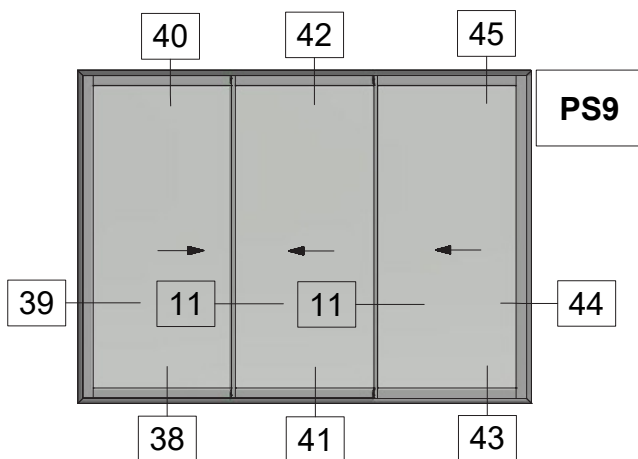
Three Sash Parallel Sliding Window 90 Degrees Cut with Narrow Interlock Τρίφυλλο Επάλληλο Συρόμενο με Κοπή 90 Μοιρών και Στενό Γάντζο
