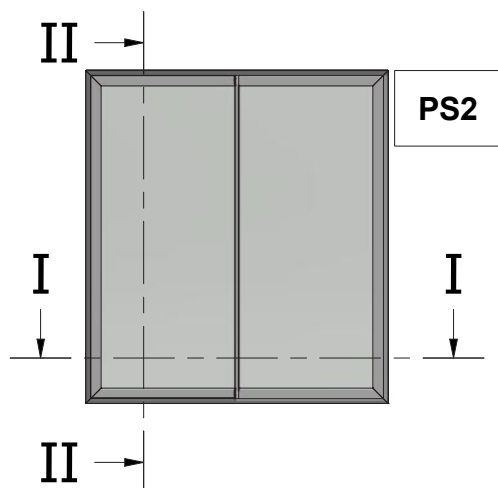
Two Sash Parallel Sliding Window 45 Degrees Cut with Narrow Interlock Δίφυλλο Επάλληλο Συρόμενο με κοπή 45 μοιρών και Στενό Γάντζο
