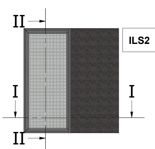
Μονόφυλλο Χωνευτό Συρόμενο με 45° κοπή με Σήτα και Παντζούρι Pocket Sliding 45° Cut with Flyscreen and Shutter
