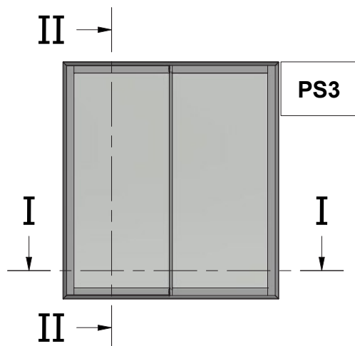
Two Sash Parallel Sliding Window 90 Degrees Cut with Narrow Interlock Δίφυλλο Επάλληλο Συρόμενο με κοπή 90 μοιρών και Στενό Γάντζο
