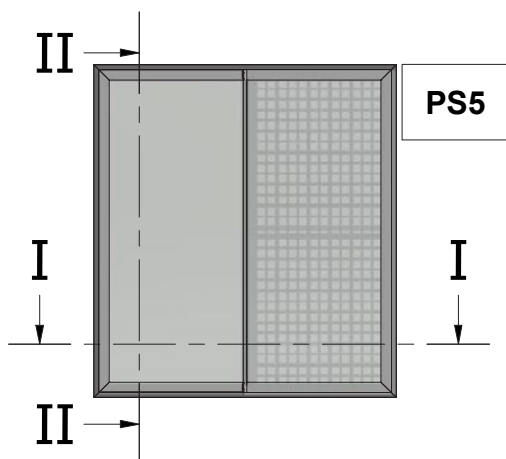
Two Sash Parallel Sliding Window 45 Degrees Cut with Narrow Interlock and Flyscreen Δίφυλλο Επάλληλο Συρόμενο με κοπή 45 μοιρών, Στενό Γάντζο και Σήτα
