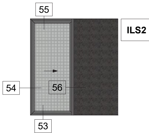
Pocket Sliding Window 45 Degrees Cut with Flyscreen and Shutter Χωνευτό Συρόμενο με κοπή 45 μοιρών Σήτα και Παντζούρι
