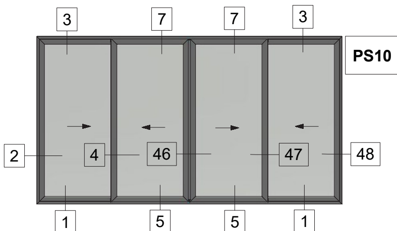
Four Sash Parallel Sliding Window 45 Degrees Cut with Meeting Stile Τετράφυλλο Επάλληλο Φιλητό Συρόμενο με κοπή 45 μοιρών
