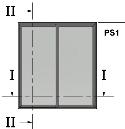
Two Sash Parallel Sliding Window 45 Degrees Cut Δίφυλλο Επάλληλο Συρόμενο με κοπή 45 μοιρών
