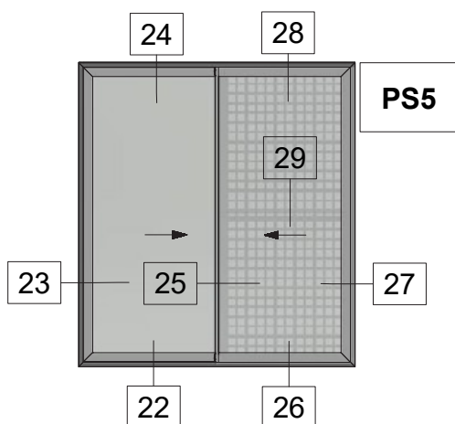
Two Sash Parallel Sliding Window 45 Degrees Cut with Narrow Interlock and Flyscreen Δίφυλλο Επάλληλο Συρόμενο με Κοπή 45 Μοιρών, Στενό Γάντζο και Σήτα
