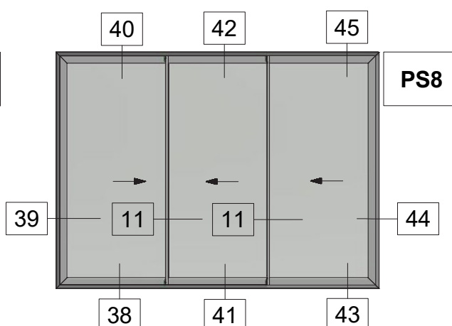
Three Sash Parallel Sliding Window 45 Degrees Cut with Narrow Interlock Τρίφυλλο Επάλληλο Συρόμενο με Κοπή 45 Μοιρών και Στενό Γάντζο
