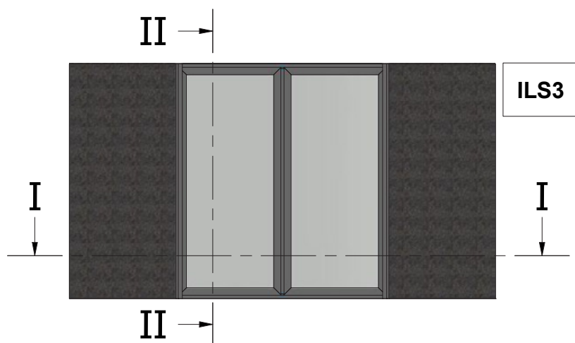
Χωνευτό Φιλητό Συρόμενο με 45° κοπή με Παντζούρι Meeting Stile Pocket Sliding 45° Cut with Shutter
