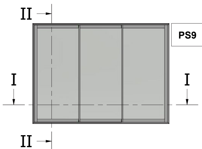
Three Sash Parallel Sliding Window 90 Degrees Cut and Narrow Interlock Τρίφυλλο Επάλληλο Συρόμενο με κοπή 90 μοιρών και Στενό Γάντζο
