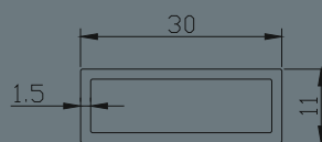
Profile 30x11mm anodised Καρέ 30x11mm
