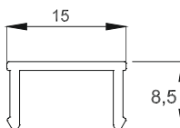
Profile for column fence Πηχάκι για κολώνα περίφραξης
