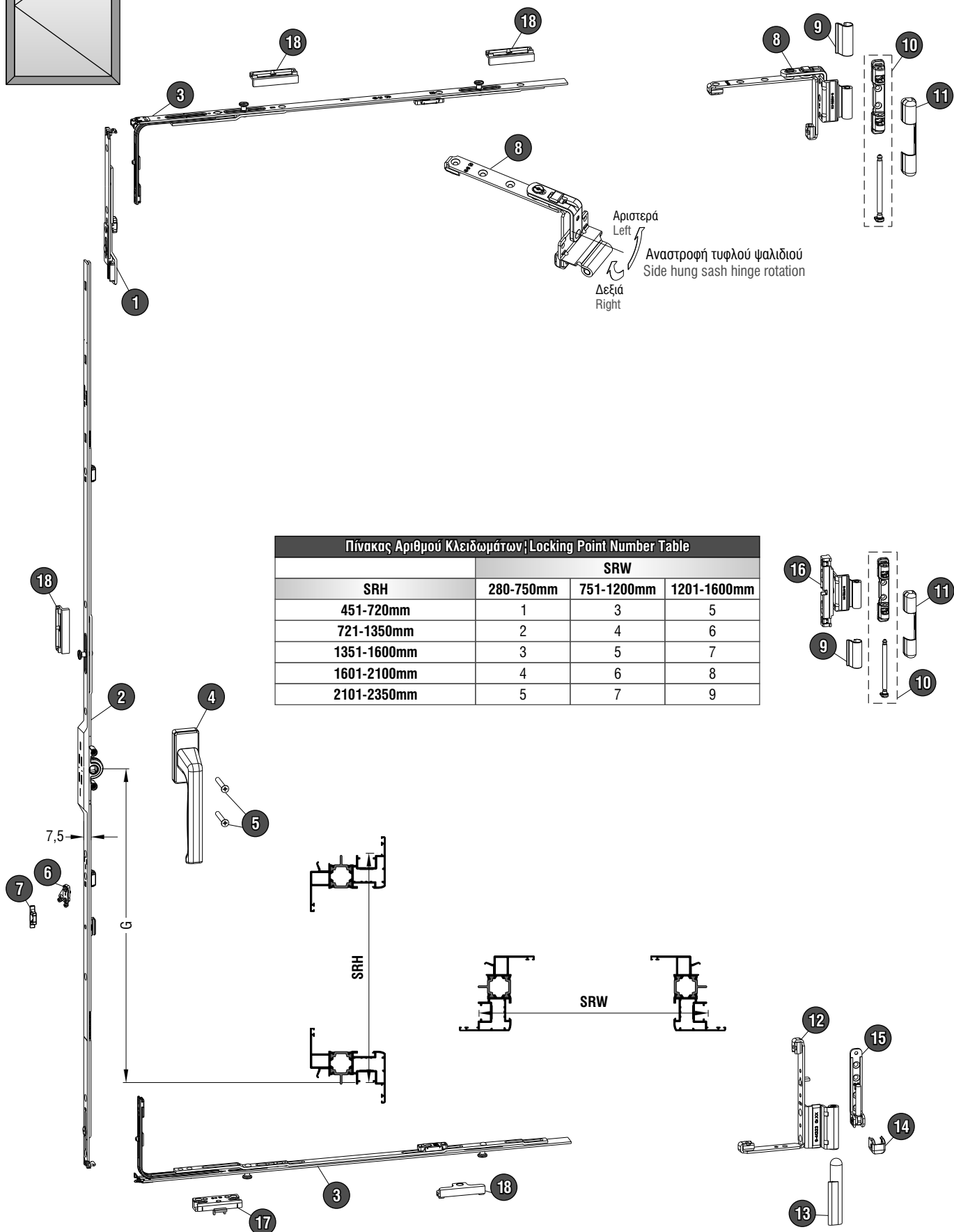
Μονόφυλλο ανοιγόμενο One sash casement window
