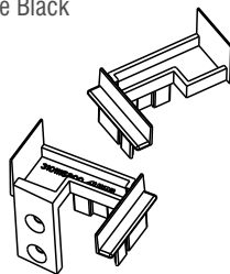
Τάπα μπινιού M11158 End cap for M11158 sash inversion profile
