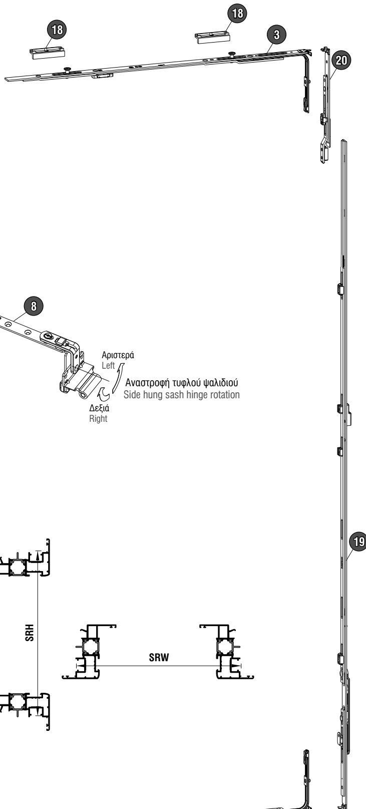
Δίφυλλο ανοιγόμενο (Δεύτερο φύλλο) Two sash casement window (Second sash)
