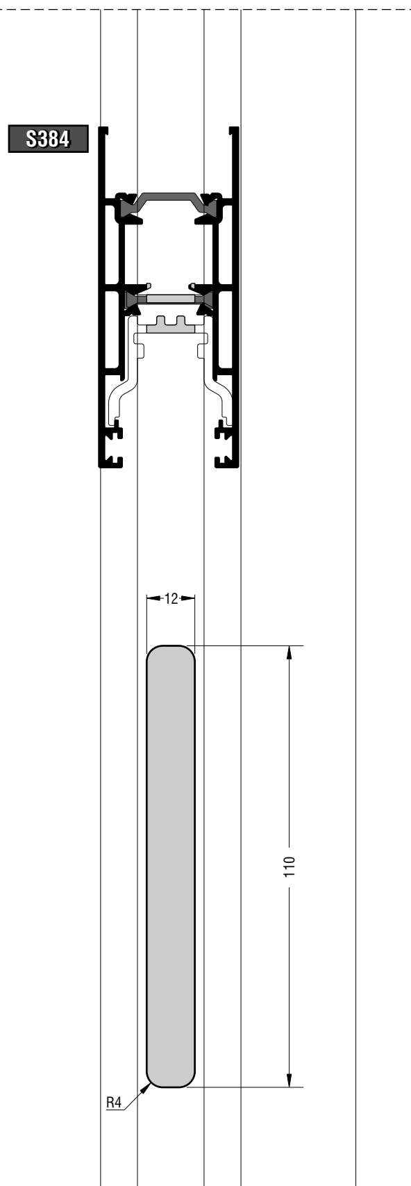
Κατεργασία κλειδαριάς Lock machining
