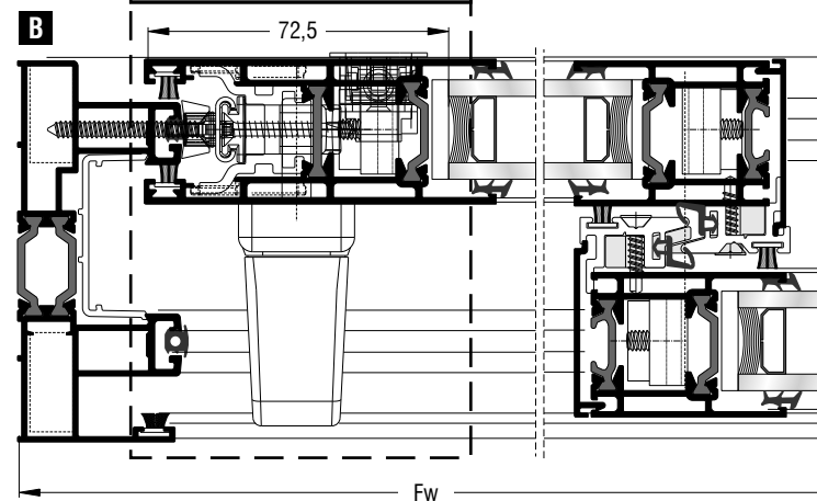
Κλειδαριά BEZAULT RIVALU BEZAULT RIVALU lock
