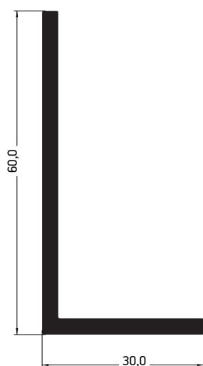
G-60x30x3 Corner profile 60x30x3 προφίλ γωνίας 60x30x3
