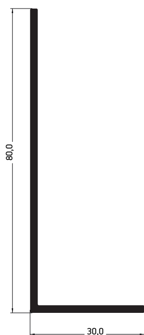
G-80x30x1,5 Corner profile 80x30x1,5 προφίλ γωνίας 80x30x1,5
