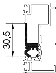
B-B ( 1 : 2 )
