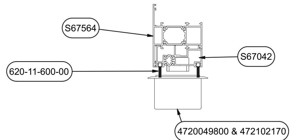
B ( 1 : 3 )
