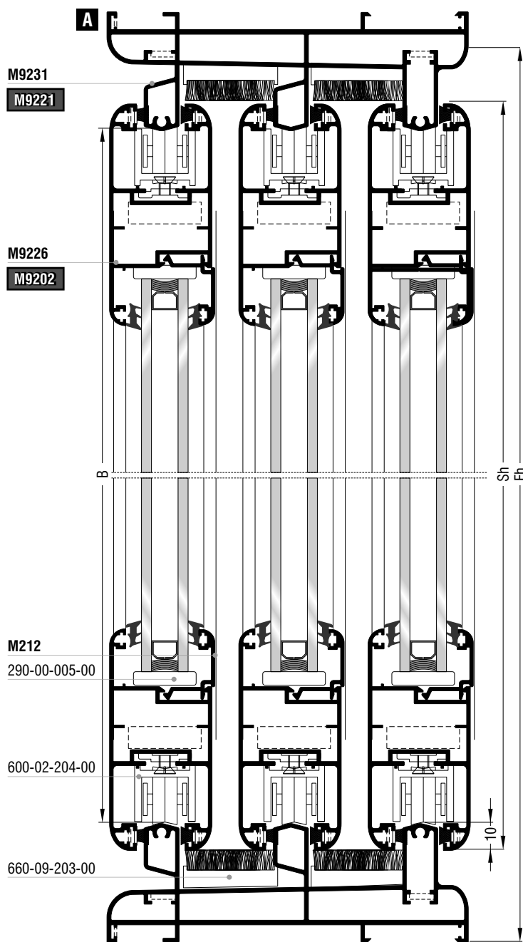
Τρίφυλλο επάλληλο συρόμενο | Three sash parallel slide
