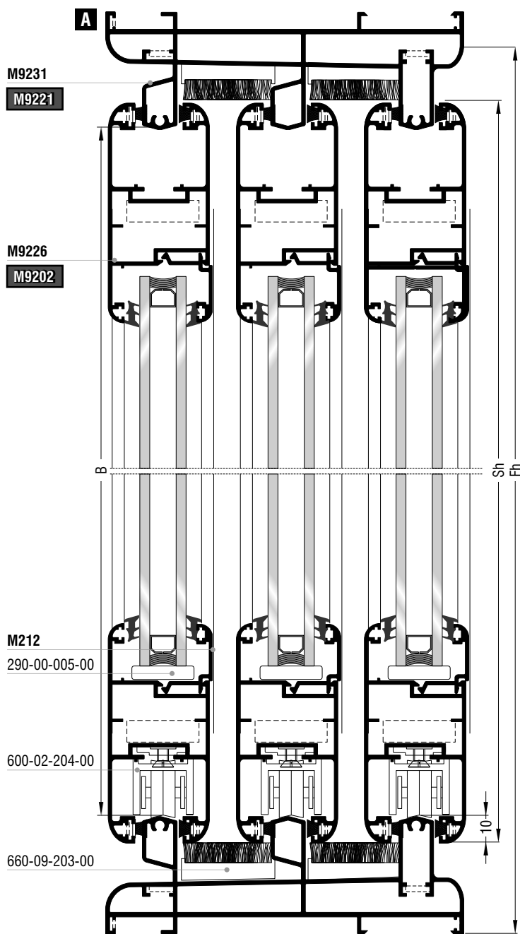
Τρίφυλλο επάλληλο συρόμενο | Three sash parallel slide
