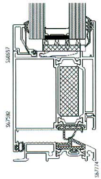
Κατακόρυφη τομή/Vertical section
