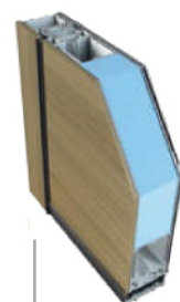
Εξωτερικό: Composite panel αλουμινίου Εσωτερικό: Ξύλο
