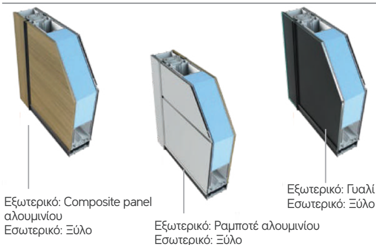
Λεπτομέρεια Ραμποτέ φύλλου με επένδυση Lamination
