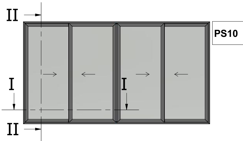
Four Sash Parallel Sliding Window with Meeting Stile 45 Degrees Cut Τετράφυλλο Φιλητό Επάλληλο Συρόμενο με κοπή 45 μοιρών
