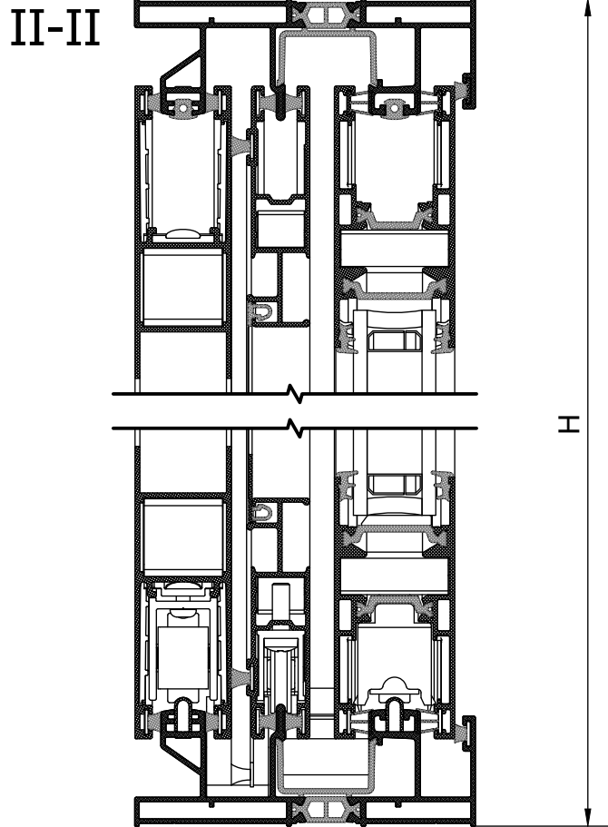
Μονόφυλλο Χωνευτό Συρόμενο με 45° κοπή με Σήτα και Παντζούρι Pocket Sliding 45° Cut with Flyscreen and Shutter
