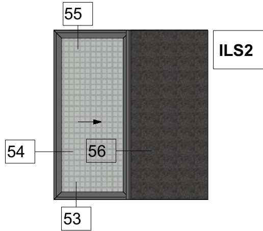
Pocket Sliding Window 45 Degrees Cut with Flyscreen and Shutter Χωνευτό Συρόμενο με κοπή 45 μοιρών Σήτα και Παντζούρι
