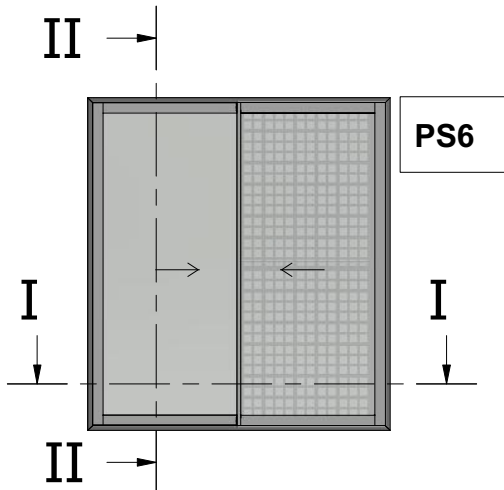
Two Sash Parallel Sliding Window 90 Degrees Cut with Narrow Interlock and Flyscreen Δίφυλλο Επτάλληλο Συρόμενο με κοπή 90 μοιρών, Στενό Γάντζο και Σήτα
