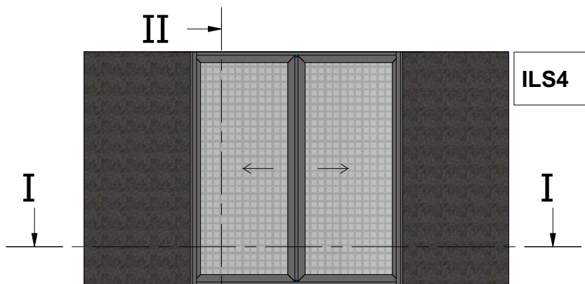
II → Χωνευτό Φιλητό Συρόμενο με 45° κοπή με Σήτα και Πανζούρι Meeting Stile Pocket Sliding 45° Cut with Flyscreen and Shutter
