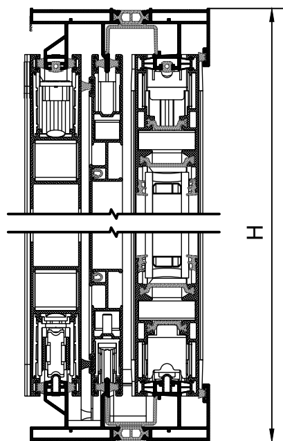
II → Χωνευτό Φιλητό Συρόμενο με 45° κοπή με Σήτα και Πανζούρι Meeting Stile Pocket Sliding 45° Cut with Flyscreen and Shutter
