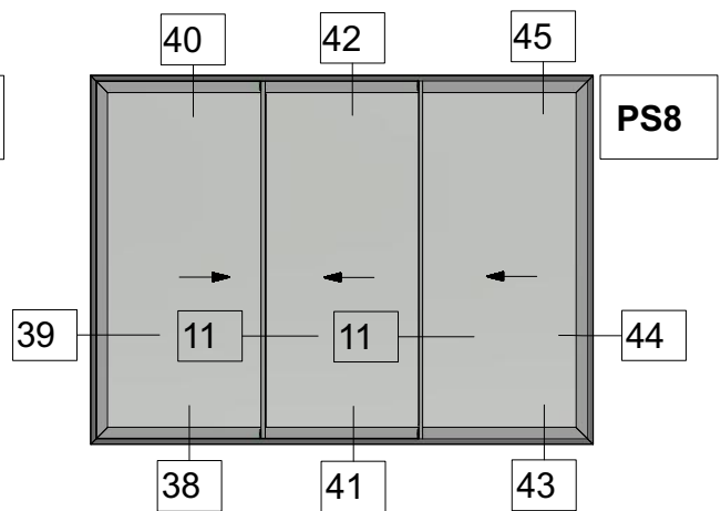
Three Sash Parallel Sliding Window 45 Degrees Cut with Narrow Interlock Τρίφυλλο Επάλληλο Συρόμενο με Κοπή 45 Μοιρών και Στενό Γάντζο
