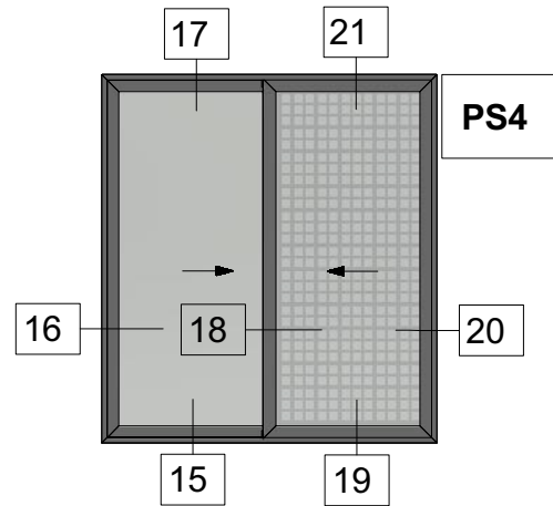
Two Sash Parallel Sliding Window 45 Degrees Cut with Flyscreen Δίφυλλο Επάλληλο Συρόμενο με κοπή 45 μοιρών και Σήτα
