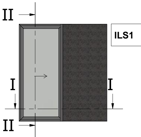
Μονόφυλλο Χωνευτό Συρόμενο με 45° κοπή με Παντζούρι Pocket Sliding 45° Cut with Shutter
