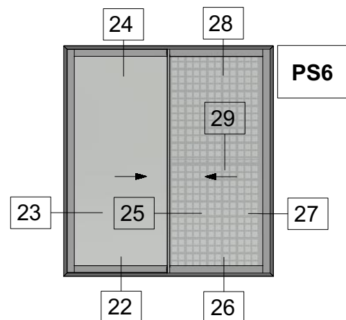
Two Sash Parallel Sliding Window 90 Degrees Cut with Narrow Interlock and Flyscreen Δίφυλλο Επάλληλο Συρόμενο με Κοπή 90 Μοιρών, Στενό Γάντζο και Σήτα
